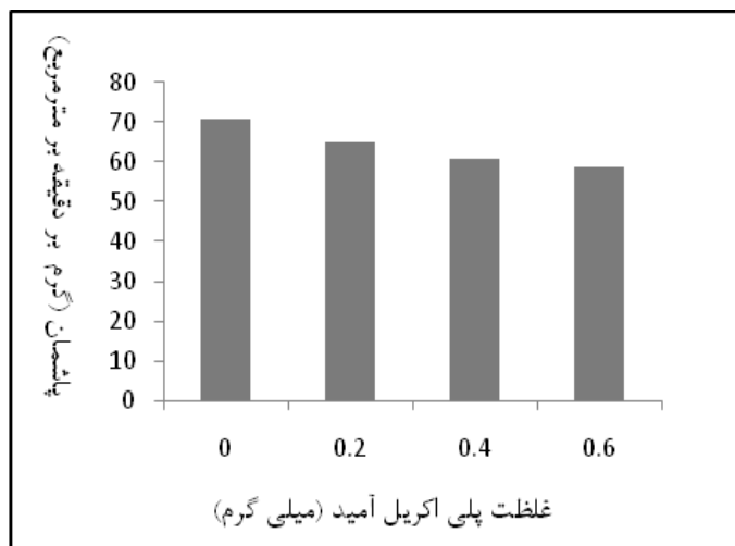
شکل ۳ - تغییرات میزان پاشمان در مقادیر مختلف پلی اکریل آمید در شدت بارندگی ۹۰ میلی متر در ساعت
