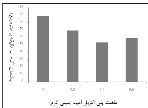
شکل ۴- تغییرات میزان پاشمان در مقادیر مختلف پلی‌اکریل‌آمید در شدت بارندگی ۱۲۰ میلی‌متر در ساعت
