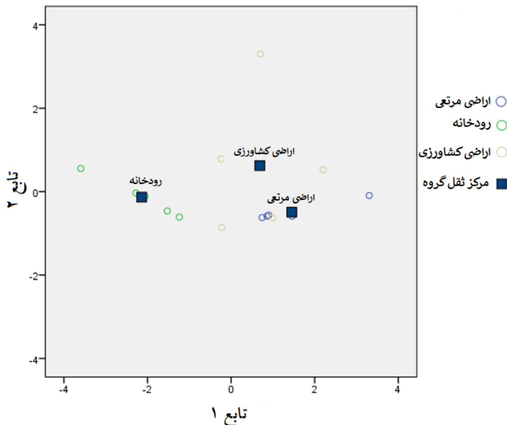
شکل ۴: تفکیک منابع از طریق توابع اول و دوم مورد استفاده در آزمون تابع تشخیص
