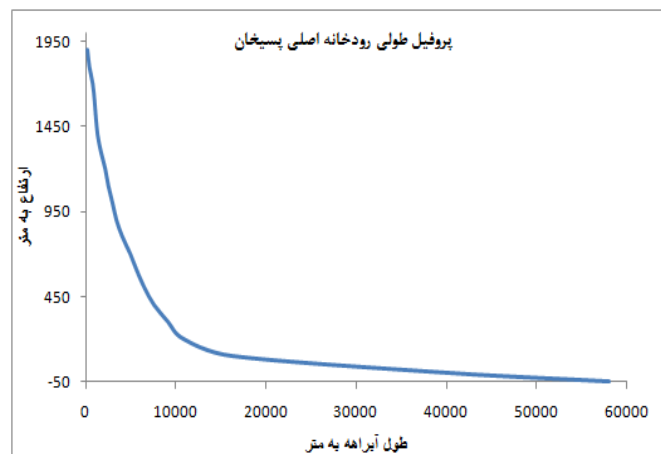
شکل ۵: پروفیل طولی شاخه چوبر - پسیخان حوضه آبخیز پسیخان
