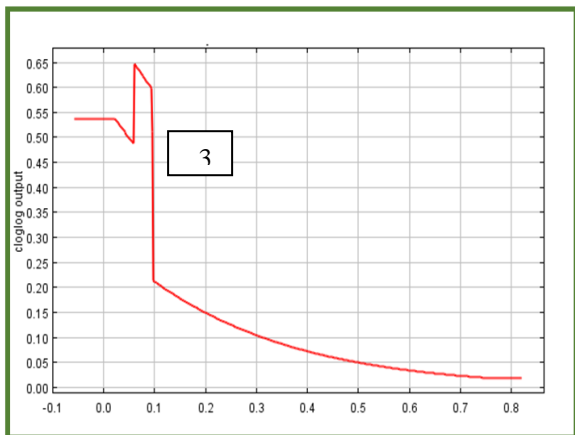
شکل ۷: منحنی پاسخ چهار شاخص با بیشترین اثرگذاری شامل: ارتفاع (۱)، کاربری اراضی (۲)، تراکم پوشش گیاهی (۳)، فاصله از آبراهه (۴) در فرسایش خندقی حوضه آبریز خسویه
