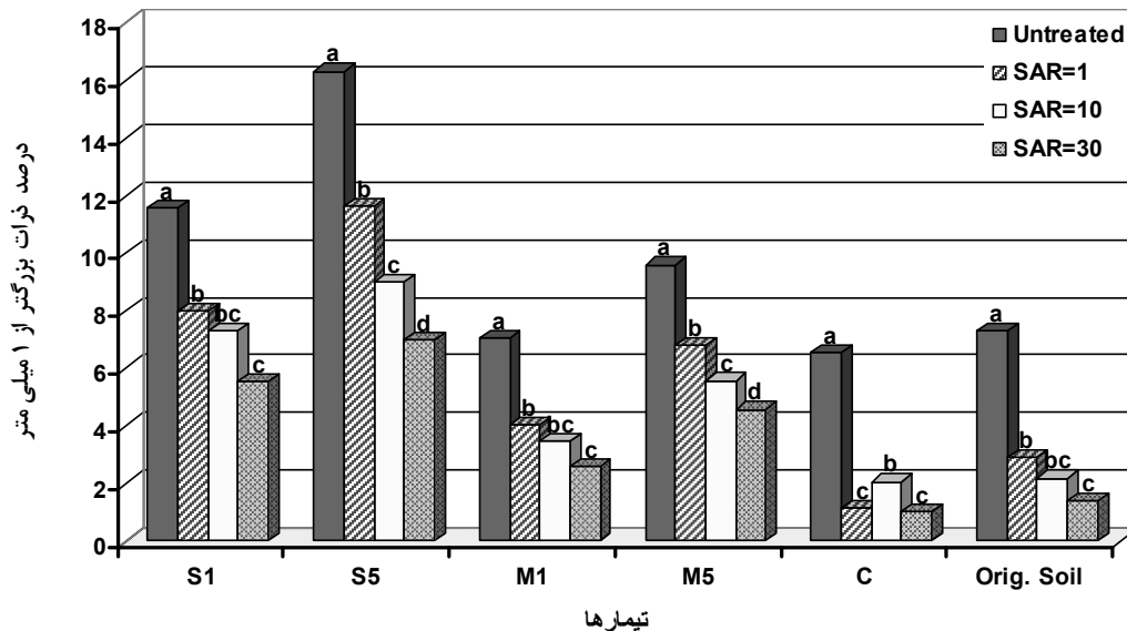
شکل ۱- درصد ذرات بزرگتر از ۱ میلی‌متر (F1) برای تیمارهای ماده آلی و آبیاری با مقادیر مختلف SAR
