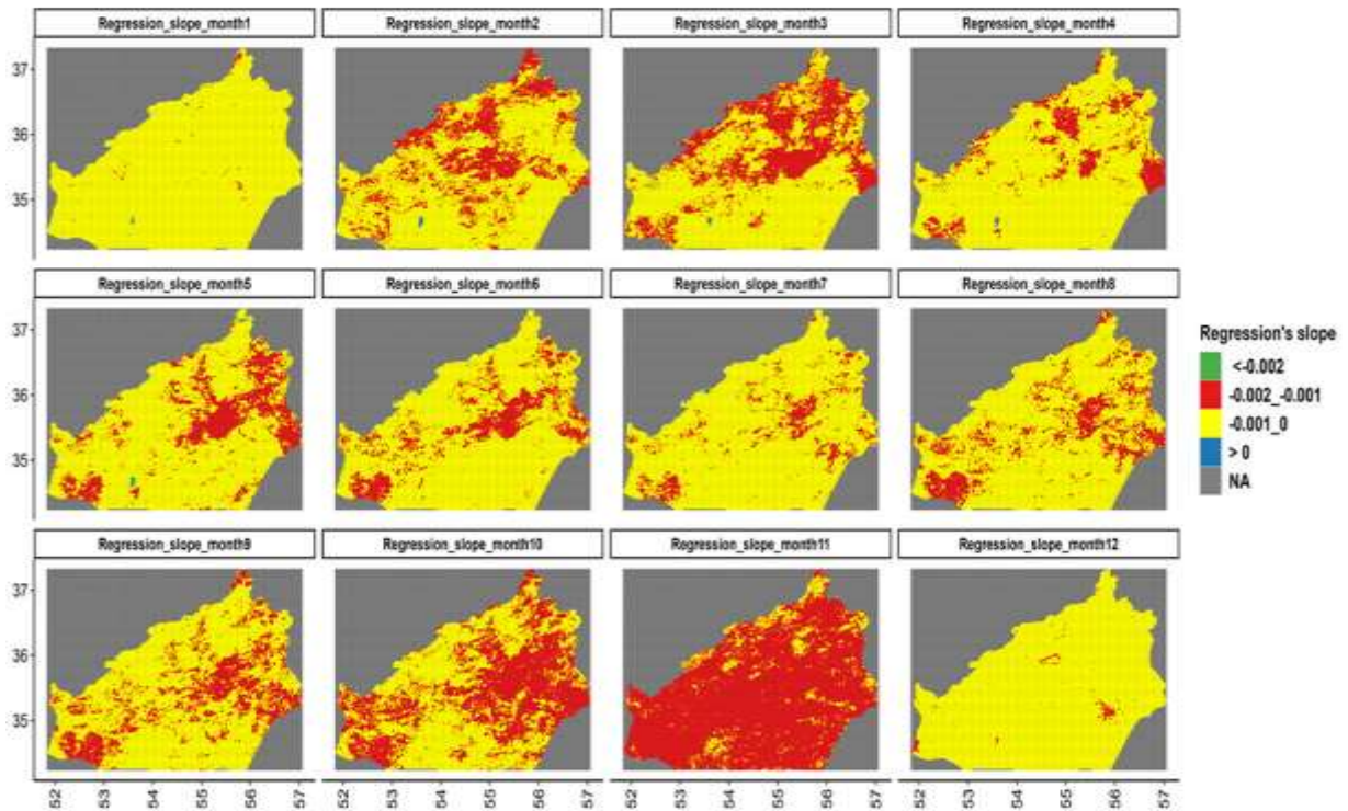
شکل ۳: شیب خط رگرسیونی سری زمانی NDVI ماهانه از سال ۲۰۰۱-۲۰۲۰
