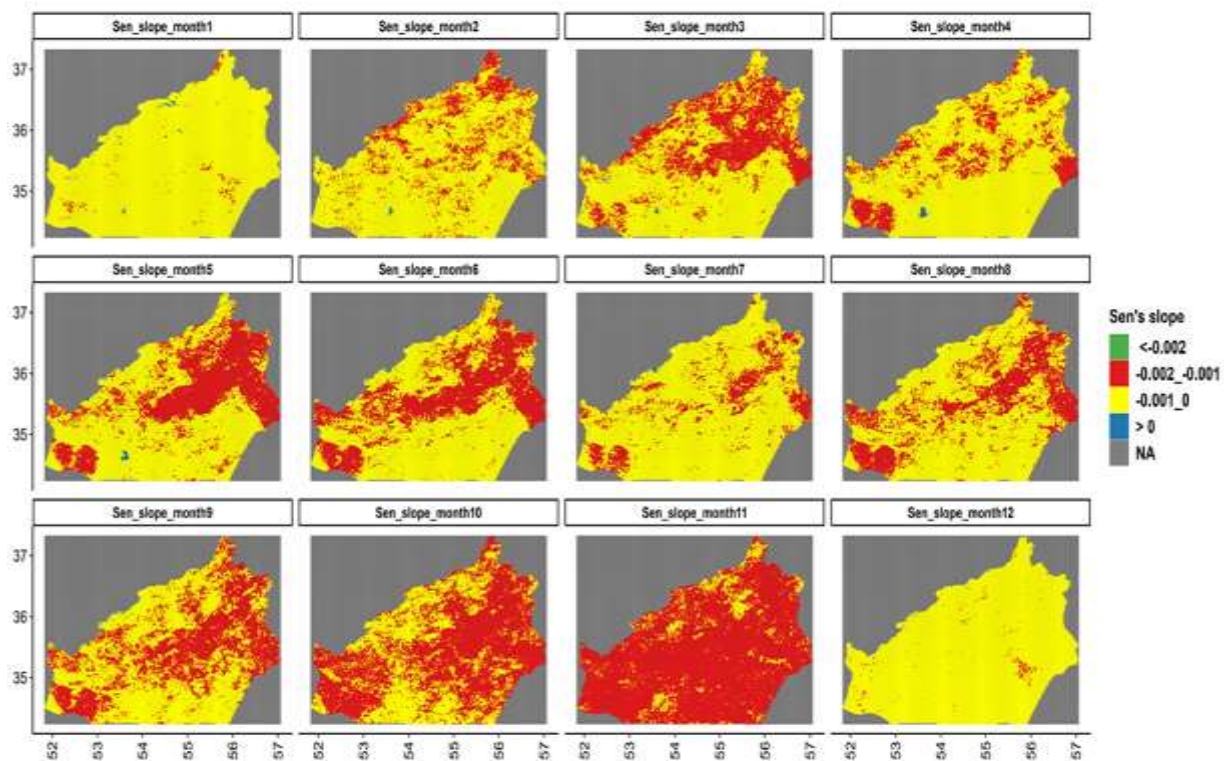
شکل ۴: تغییرات شیب خط تخمین گر سن در سری زمانی NDVI در هر ماه طی سال‌های ۲۰۲۰-۲۰۱۱
