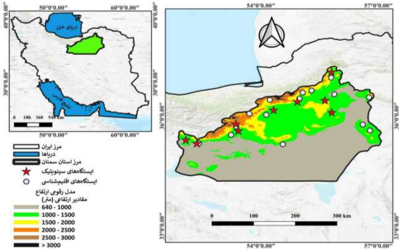
شکل ۱: موقعیت قرارگیری استان سمنان در ایران و شماتیک تغییرات ارتفاعی و پراکنش ایستگاه‌های سینوپتیک و اقلیم‌شناسی در استان سمنان
