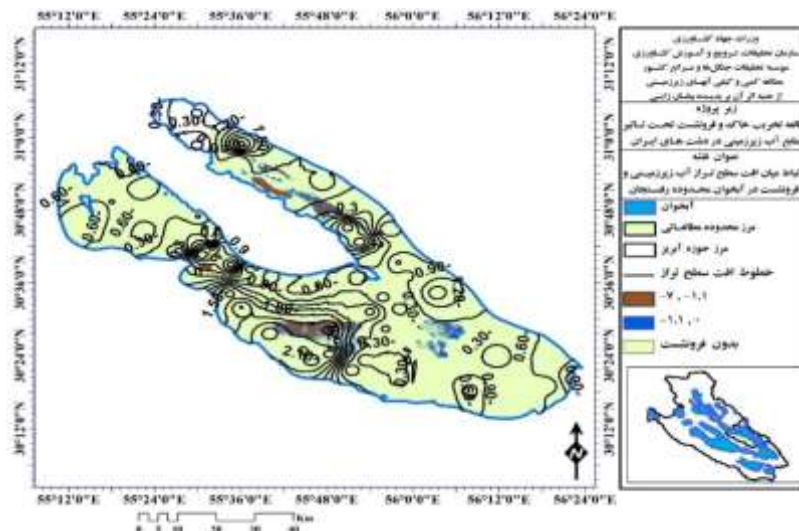
شکل ۴: ارتباط میان افت سطح تراز آب زیرزمینی و نواحی دارای فرونشست در سال‌های آبی ۱۳۹۴-۹۵ و ۱۳۹۵-۹۶
