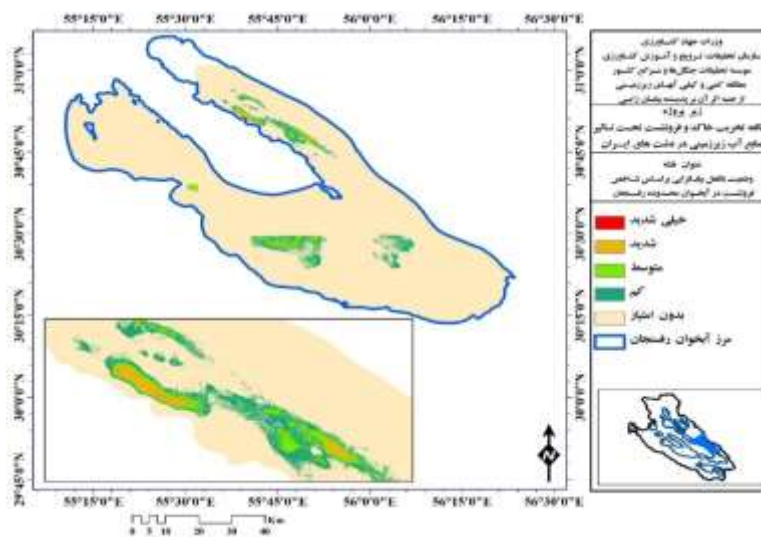
شکل ۳: وضعیت بالفعل بیابان‌زایی بر اساس شاخص فرونشست در آبخوان رفسنجان- سال آبی ۱۳۹۴-۹۵
