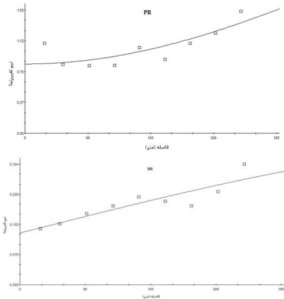
شکل ۳: نیم تغییرناها (نقاط) و مدل‌های برازش شده (خطوط) مقاومت فروروی (PR) و مقاومت برشی (SS) خاک.
