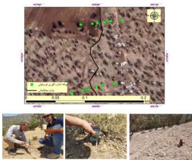
شکل ۲: اندازه‌گیری میدانی فرسایش و رسوب به کمک پیکه‌های فرسایشی در منطقه
