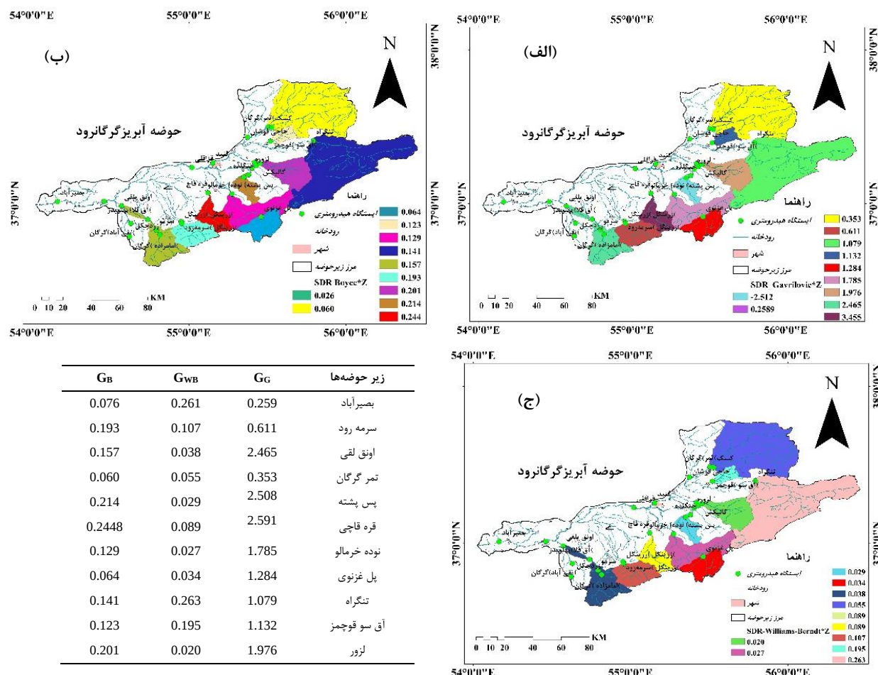
شکل ۷- نقشه بازده رسوب (G) در زیرحوضه‌های مورد مطالعه حوضه که توسط مدل EPM بر اساس معادله نسبت تحویل رسوب (الف) گاوریلیج،
