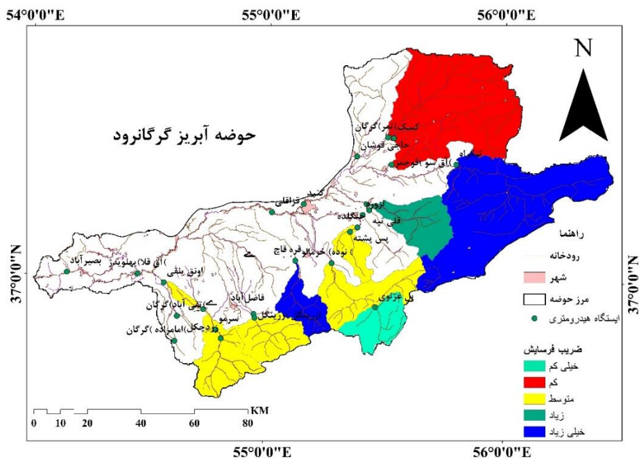
شکل ۵- نقشه شدت فرسایش (Z) در زیرحوضه‌های حوضه آبریز گرگانرود
