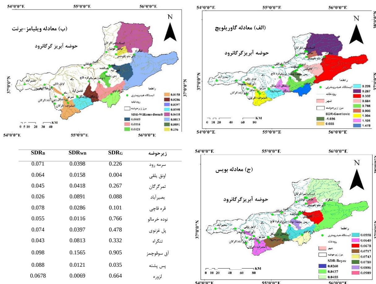
شکل ۶- نقشه‌های نسبت تحویل رسوب (SDR) زیرحوضه‌های مورد مطالعه که بر اساس سه معادله (الف) گاوریلویج SDR G ، (ب) ویلیامز-برنت SDR B و (ج) بویس SDR WB
