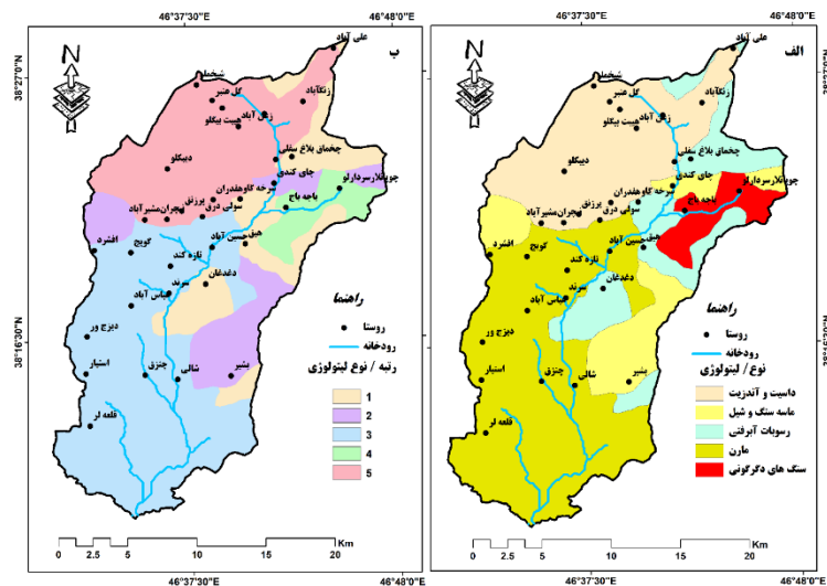
شکل ۷: الف) نقشه لیتولوژی. ب) نقشه وزنی لیتولوژی حوزه آبریز سرنندچای
