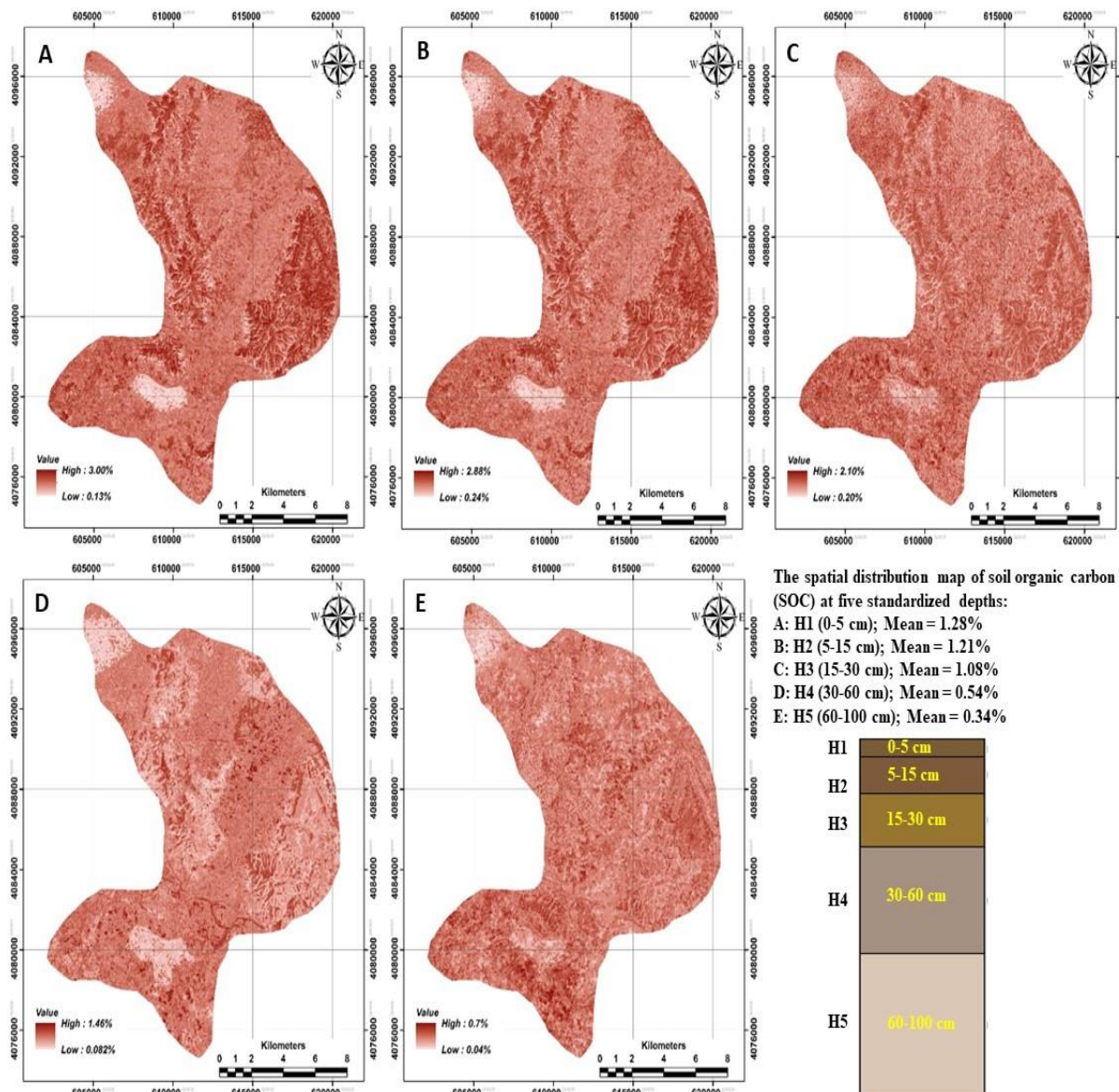
شکل ۲: نقشه پراکنش مکانی کربن آلی خاک در عمق‌های استاندارد شده
