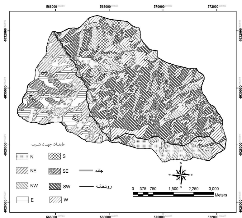
شکل ۵ - نقشه جهت دامنه حوضه مورد مطالعه
