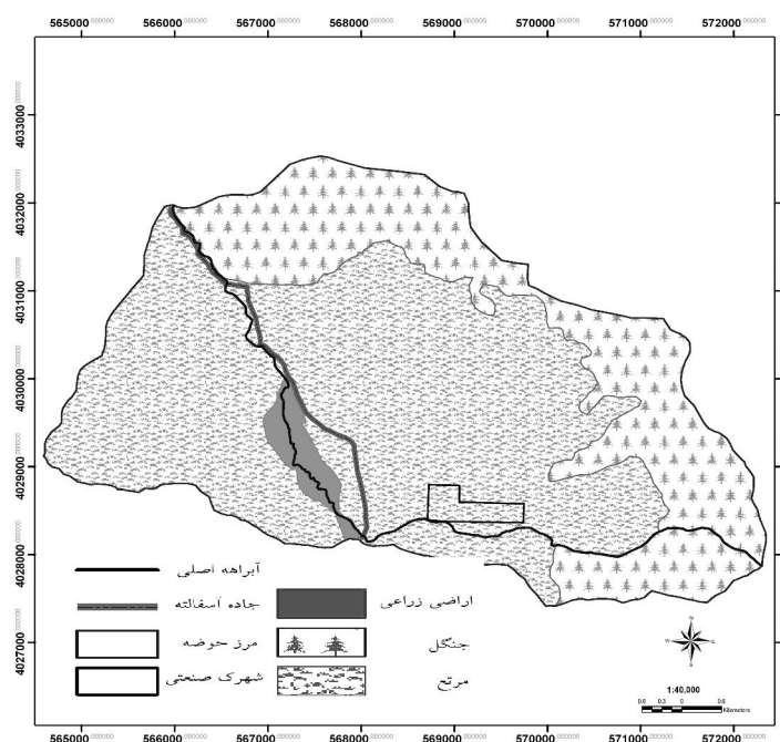
شکل ۳ - نقشه‌ی پوشش گیاهی حوضه‌ی مورد مطالعه
