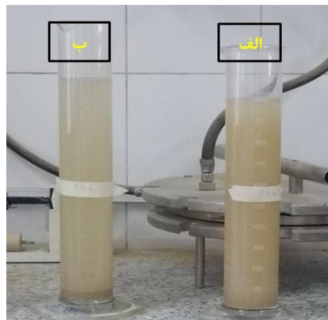
شکل ۸: نمایی از آزمایش هیدرومتری دوگانه، الف) پراکنش ذرات در حالت استفاده از ماده شیمیایی پراکنده ساز (محلول هگزا متافسفات سدیم)، ب) پراکنش ذرات در حالت بدون استفاده از ماده شیمیایی پراکنده ساز (فقط محلول آب مقطر) در قرائت زمانی یکسان
