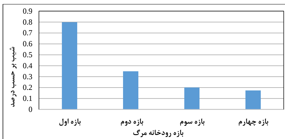
شکل ۱۵: میزان شیب بستر بازه‌های مختلف رودخانه مرگ بر حسب درصد
