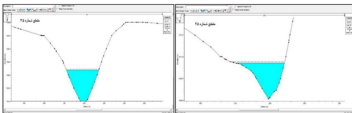
شکل ۱۰: مقاطع انتخابی رودخانه مرگ در بازه اول
