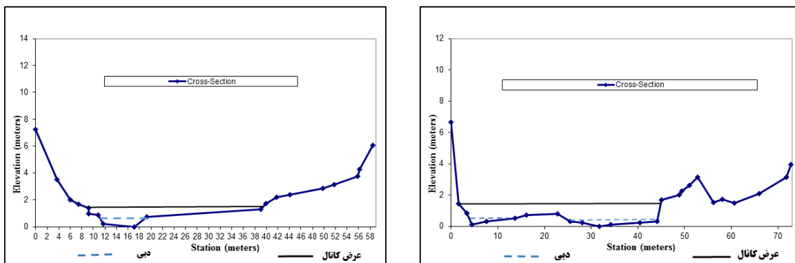
شکل ۱۲: نیمرخ عرضی رودخانه در بازه هشت
