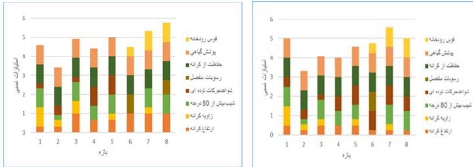
شکل ۱۶: امتیاز نسبی عوامل مؤثر در فرسایش کرانه رودخانه قلعه رودخان در کرانه راست (نمودار سمت راست) و کرانه چپ (نمودار
