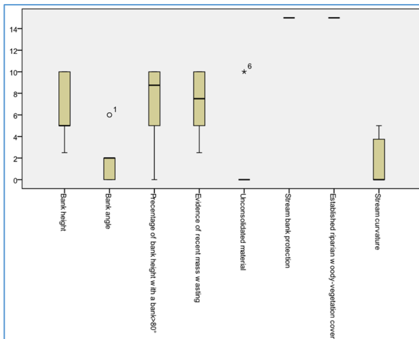
شکل ۱۷: نمودار باکس پلات امتیازهای هر یک از متغیرها به صورت مجزا برای کرانه چپ در شاخص پتانسیل فرسایش کناره رودخانه پایداری کانال
