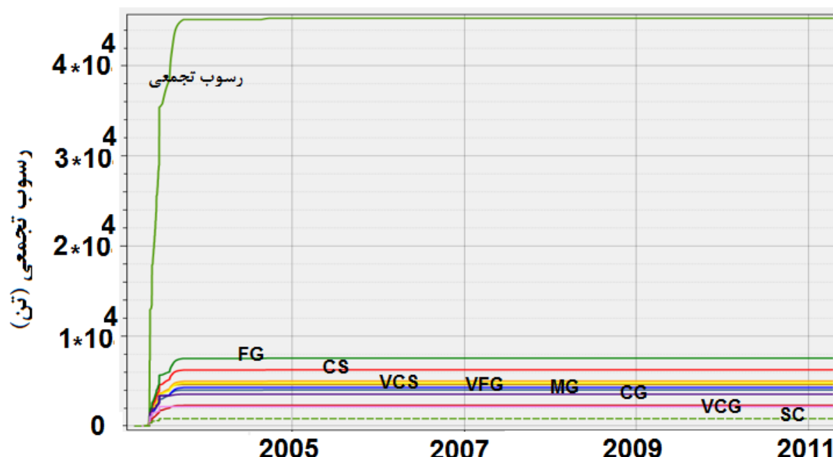
شکل ۹: مشخصات رسوبات ورودی برای دانه‌بندی‌های مختلف در مقطع عرضی شماره ۲۵۸۷۸/۲۹
