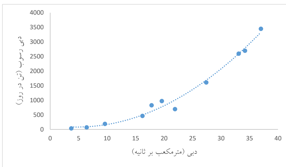
شکل ۳: منحنی سنج
