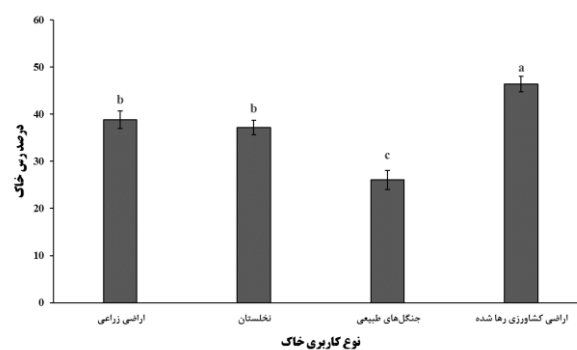
شکل ۲: الف) توزیع کلاس بافتی خاک‌های مورد مطالعه در مثلث بافت خاک، ب) تأثیر نوع کاربری‌های مورد مطالعه بر درصد ذرات رس، ج) سیلت، د) شن و هـ) سطح ویژه خاک
