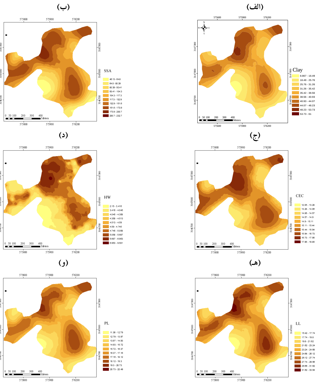
شکل ۵: الف) نقشه کریجینگ درصد رس خاک، ب) سطح ویژه، ج) ظرفیت تبادل کاتیونی، د) رطوبت هیگروسکوپی، ه) حد روانی، و) حد خمیری خاک در منطقه مورد مطالعه
