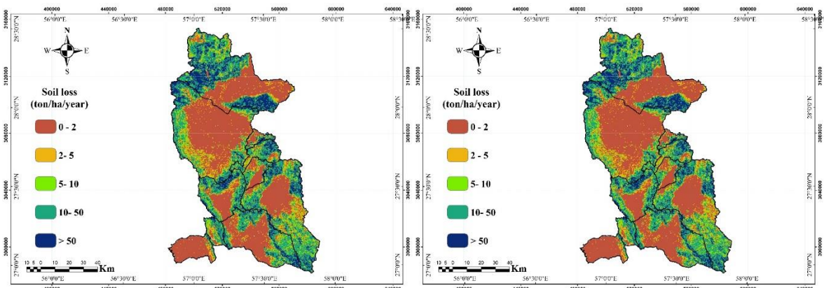
شکل ۲۵: فرسایش حوضه میناب ۲۰۴۰
