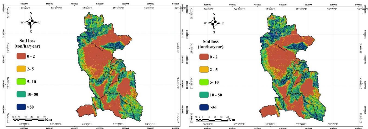
شکل ۲۱: فرسایش حوضه میناب ۲۰۴۰
