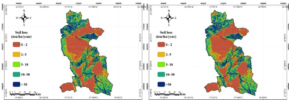
شکل ۲۳: فرسایش حوضه میناب ۲۰۴۰
