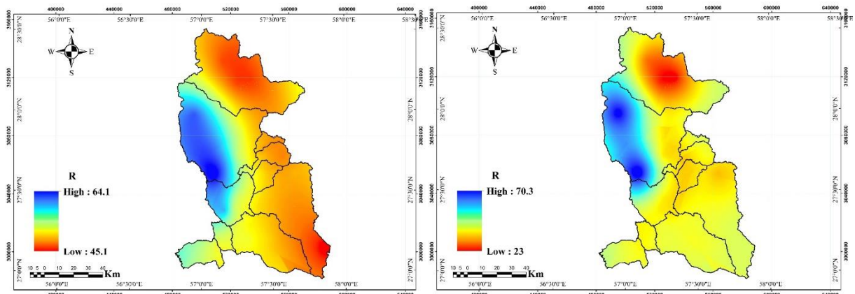
شکل ۸: لایه فرساینده باران در دوره ۲۰۱۰-۲۰۰۰
