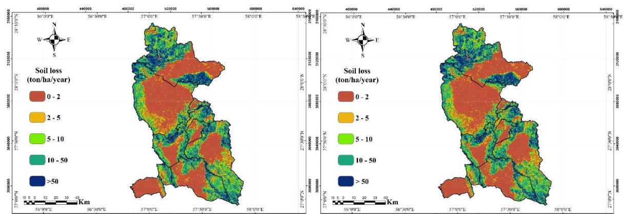
شکل ۱۰: فرسایش حوضه میناب در دوره ۲۰۱۰-۲۰۰۰
