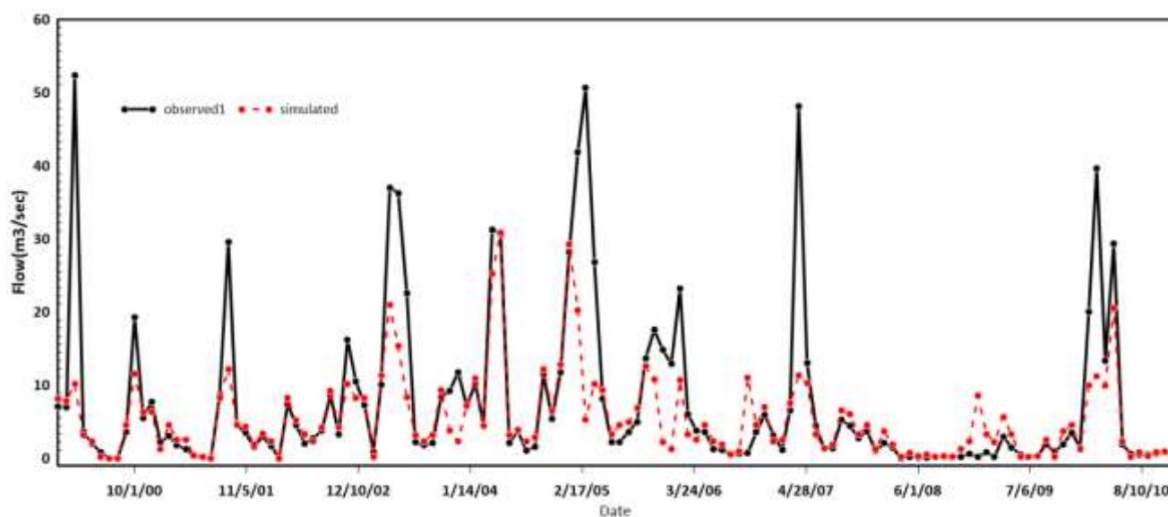
نمودار ۳: نتایج واسنجی دوره دوم مدل SWAT با استفاده از الگوریتم SUFI-2
