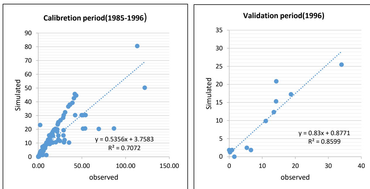
نمودار ۲: نتایج همبستگی بین رواناب مشاهده شده و شبیه‌سازی شده در مرحله کالیبراسیون و اعتبارسنجی دوره اول مدل SWAT با استفاده از الگوریتم SUFI-2
