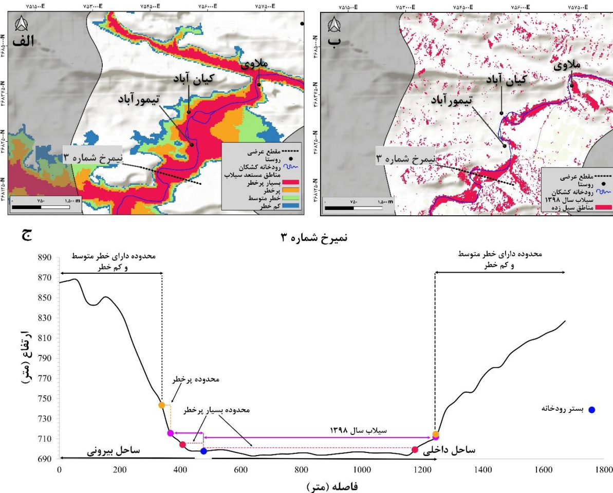
شکل ۷: الف) نمای بزرگ شده نقشه مناطق مستعد سیلاب با مدل HAND، ب) نمای بزرگ شده مناطق سیل‌زده با استفاده از تصاویر راداری، ج)
