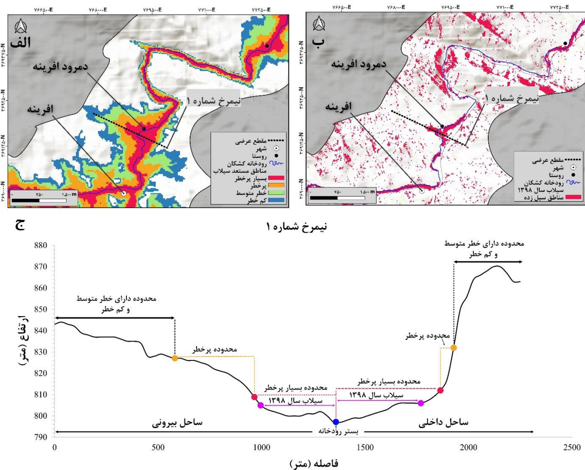
شکل ۱: الف) نمای بزرگ شده نقشه مناطق مستعد سیلاب با مدل HAND، ب) نمای بزرگ شده مناطق سیل‌زده با استفاده از تصاویر راداری، ج)
