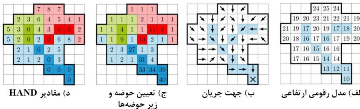
شکل ۲: نحوه عملکرد مدل HAND در تعیین مناطق مستعد سیلاب (برگرفته شده از Rebolho و همکاران (۲۰۱۸))
