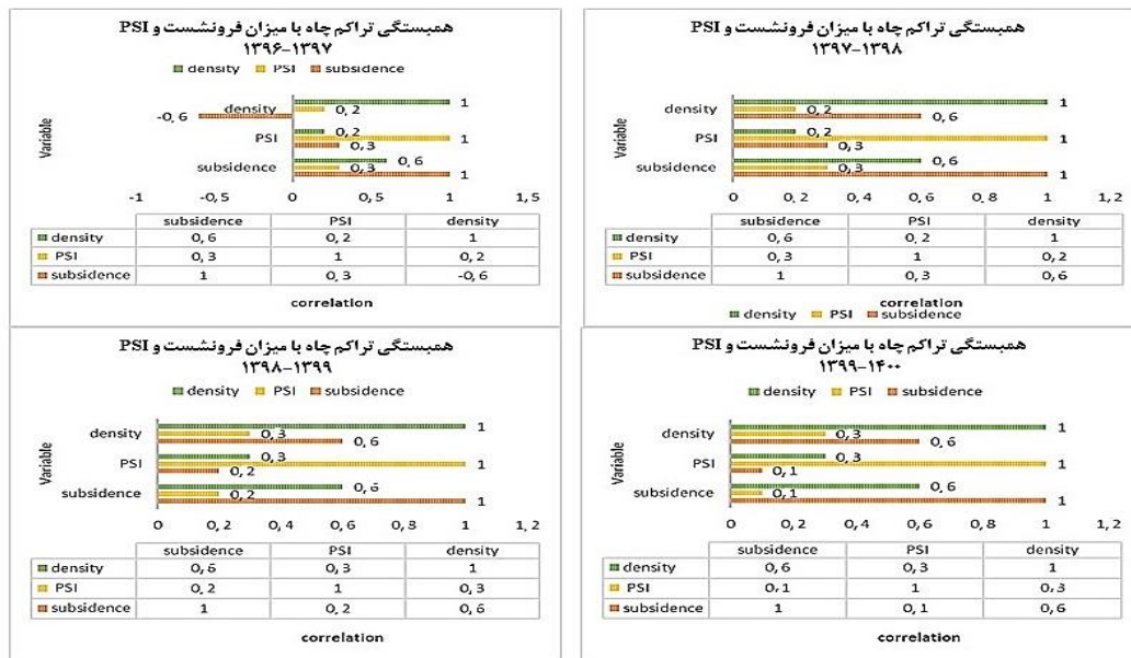
شکل ۸: همبستگی تراکم چاه‌ها با میزان فرونشست و شاخص خشکسالی آب زیرزمینی (PSI)
