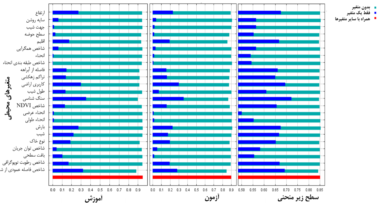
شکل ۷- نتایج تحلیل جک نایف در بررسی سهم متغیرها در تهیه نقشه حساسیت به فرسایش خندقی
