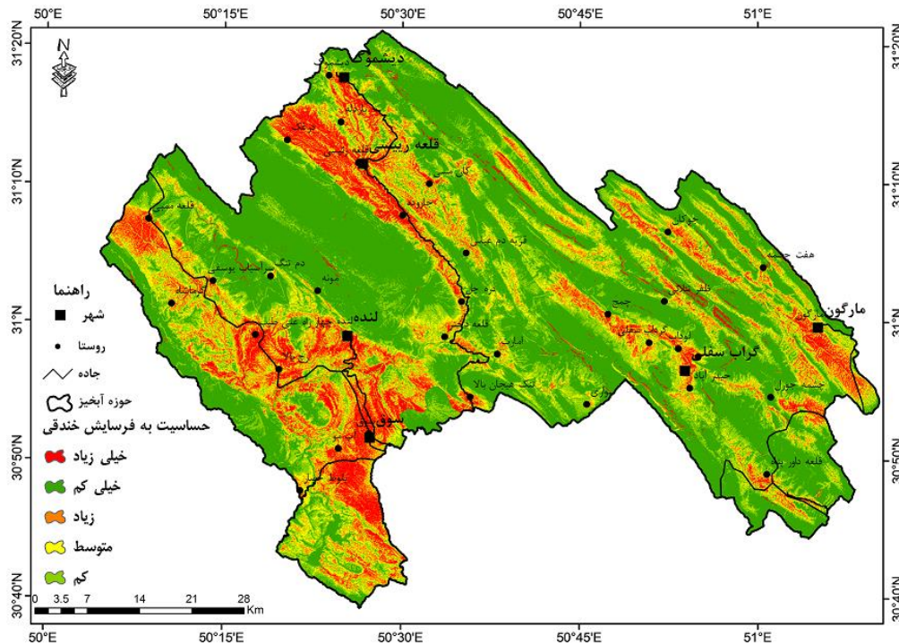
شکل ۴- پهنه بندی حساسیت به فرسایش خندقی در مدل حداکثر آنترویی
