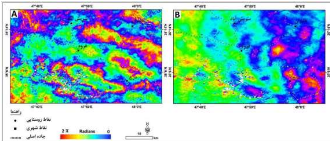
شکل ۳: نقشه‌ها اینترفروگرام (A) ۲۰۱۸/۰۱/۲۴-۲۴/۰۲/۱۷ تا ۲۰۱۸/۰۱/۲۷-۲۰۱۹/۱۱/۲۰ (B)
