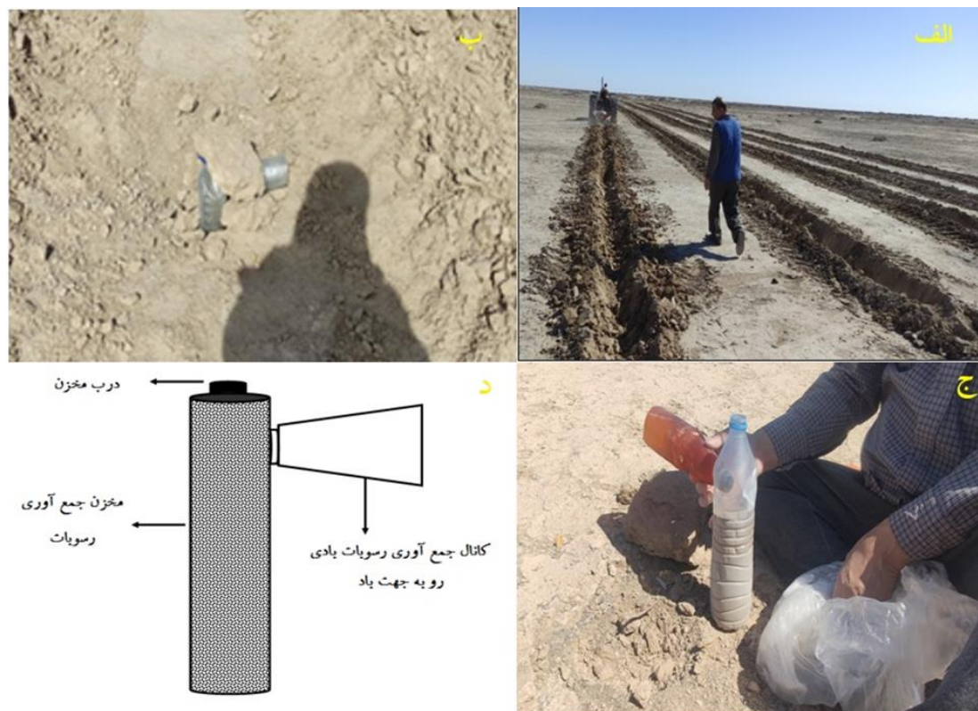
شکل ۲: نمایشی از فرآیند اجرای طرح در منطقه کاروانسرای شهرستان نيمروز، الف) نمایشی از نحوه احداث فاروها، ب) نمایشی از تله رسوبگیر نصب شده در محدوده اجرای طرح، ج) نمایشی از میزان رسوبات به دام افتاده در تله‌های رسوبگیر، د) شکل شماتیک از اجزای تشکیل دهنده تله رسوبگیر مورد استفاده در پژوهش حاضر.
