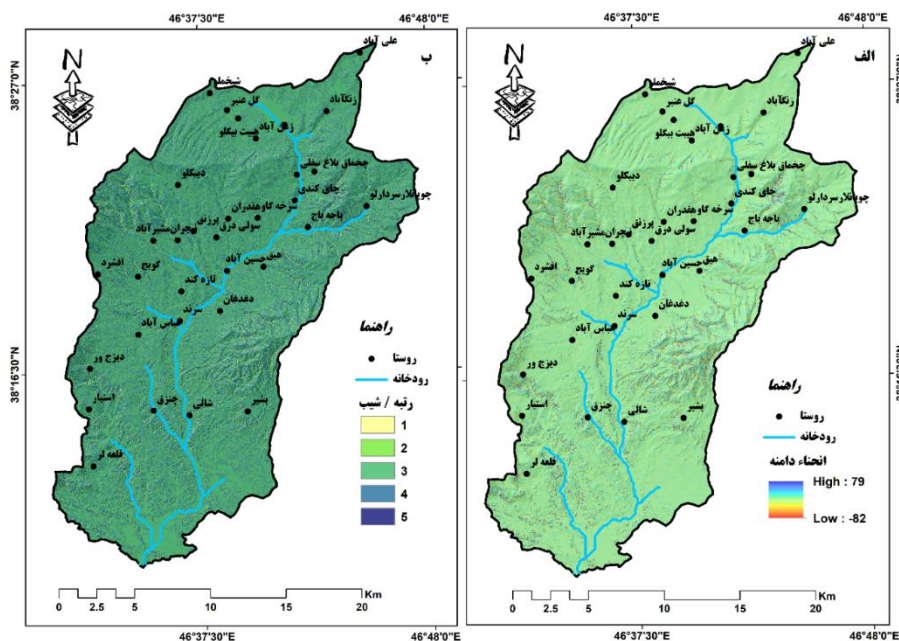
شکل ۵: الف) نقشه انحنای دامنه. ب) نقشه وزنی انحنای دامنه حوضه آبریز سرنندچای
