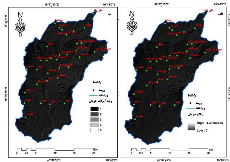
شکل ۴: الف) نقشه تراکم جریان (ب) نقشه وزنی تراکم جریان حوضه آبریز سرنندچای
