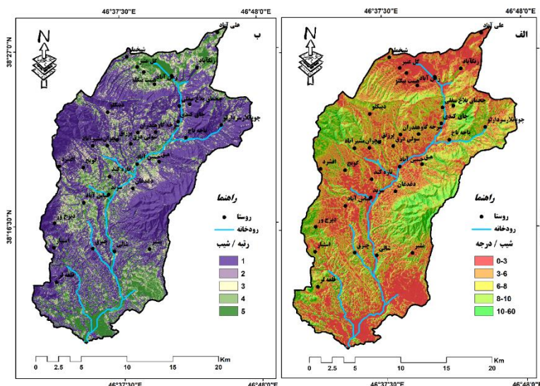
شکل ۳: الف) نقشه شیب؛ ب) نقشه لایه وزن‌دار شیب حوزه آبریز سرنده‌چای
