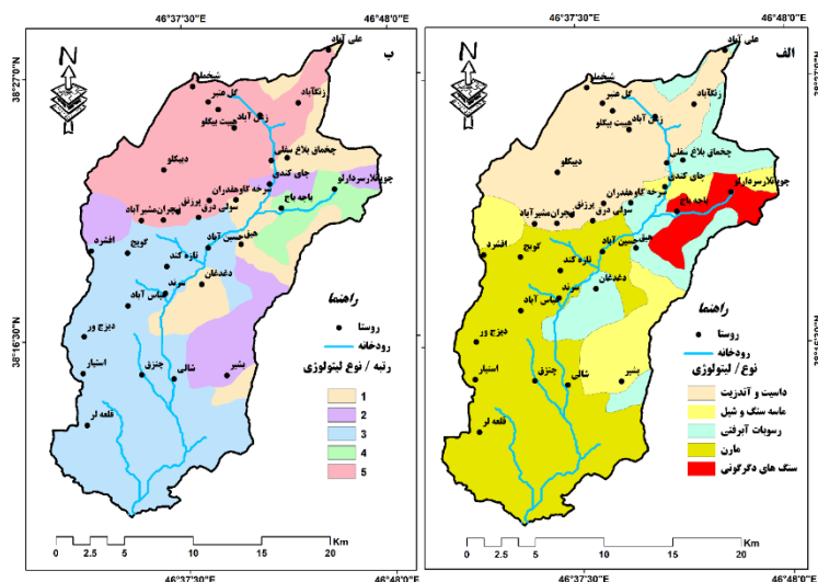
شکل ۷: الف) نقشه لیتولوژی. ب) نقشه وزنی لیتولوژی حوزه آبریز سرندهای
