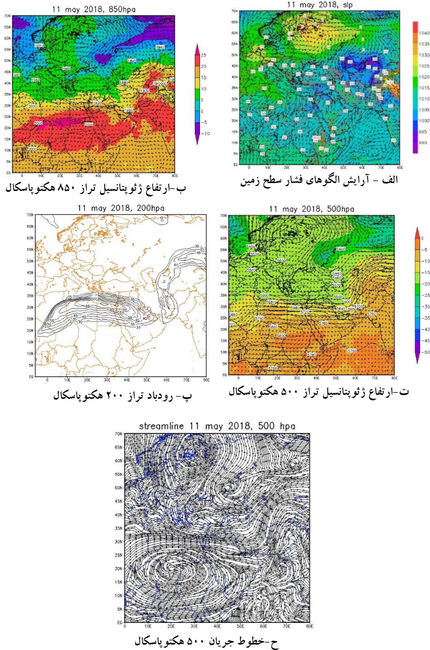
شکل ۵: نقشه‌های سطوح مختلف جو ساعت صفر UTC روز ۱۱ می ۲۰۱۸ (دما برحسب درجه سلسیوس، فشار برحسب هکتوپاسکال و ارتفاع برحسب متر)
