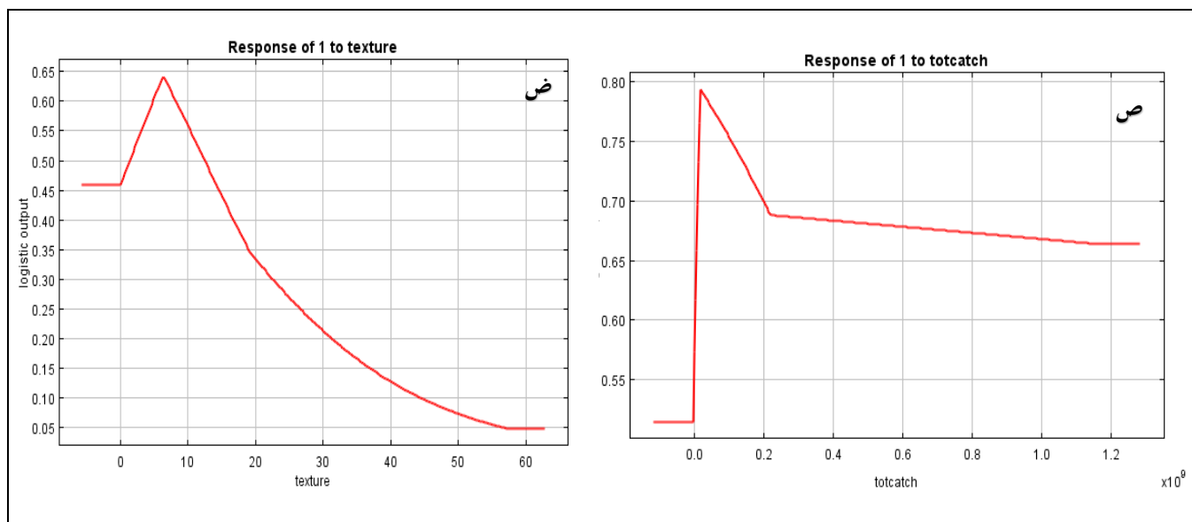
شکل ۶: منحنی پاسخ آستانه‌های حساسیت فرسایش خندقی ذ: انحنا کلی ر: نمودار شاخص تفاضل پوشش گیاهی ز: نمودار پاسخ شاخص بارش ژ: نمودار پاسخ شاخص پروفیل طولی س: نمودار پاسخ شاخص شیب ش: نمودار پاسخ شاخص خاک ص: نمودار پاسخ شاخص مساحت حوضه ض: نمودار پاسخ شاخص بافت
