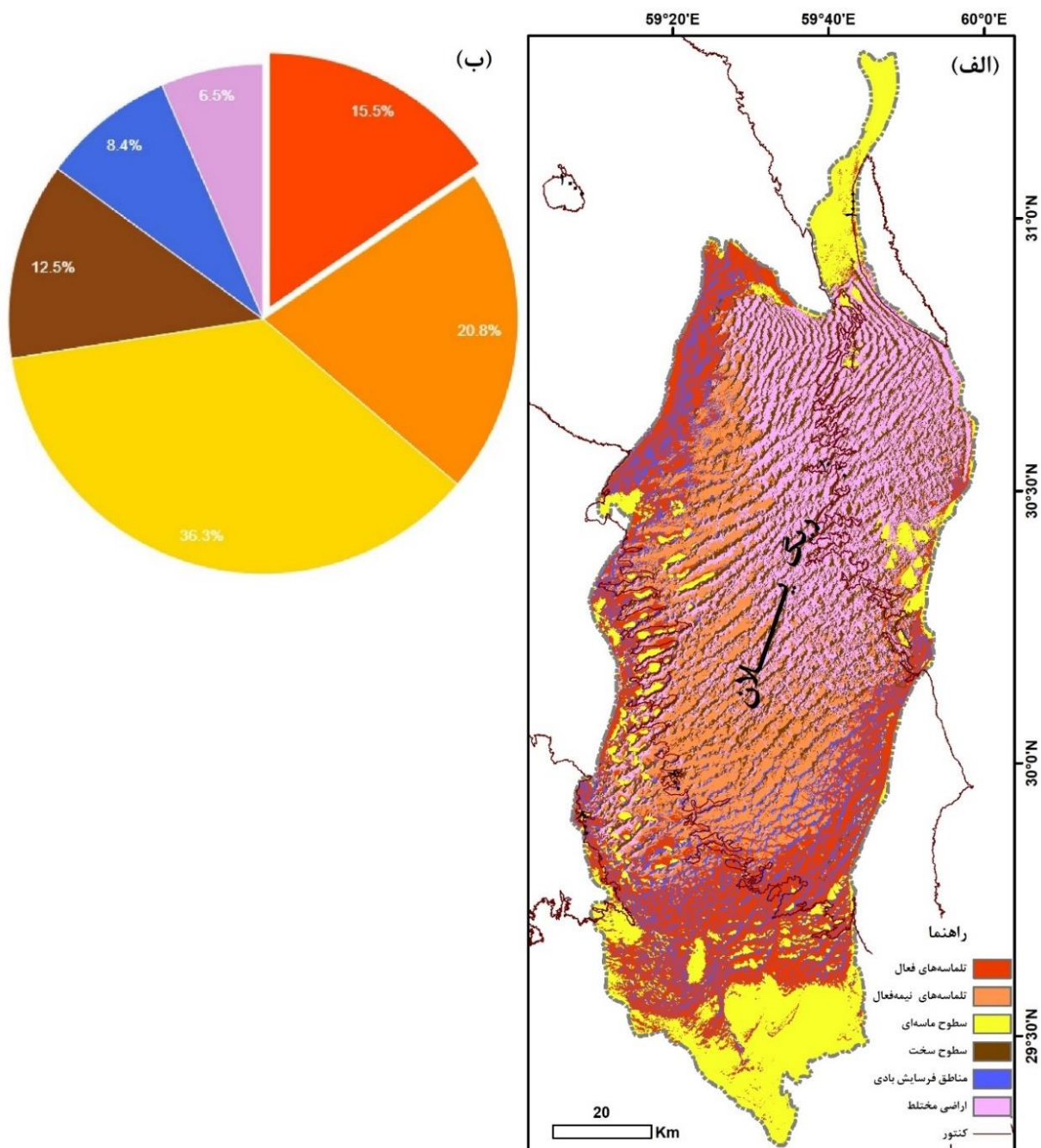
شکل ۳ توزیع فایه‌ی واحدهای همگن مورفودینامیک در ریگ یلان
