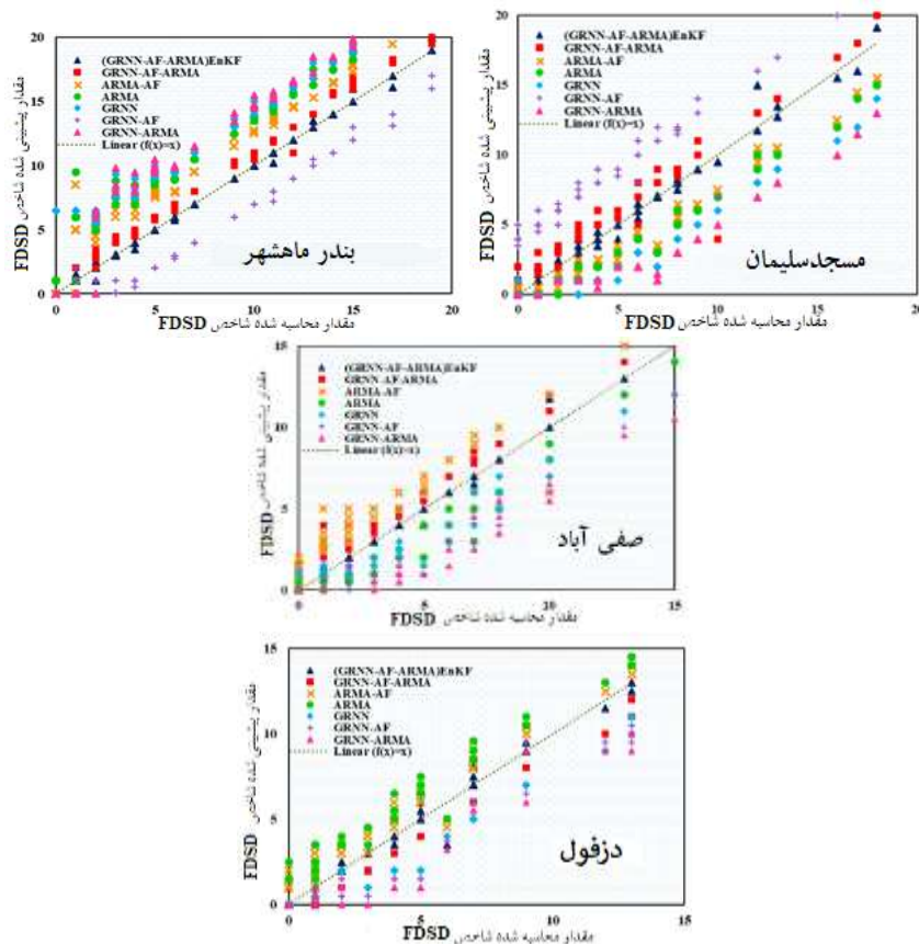
شکل ۴: مقایسه مقادیر مشاهده شده و پیش‌بینی شده شاخص FDSD با استفاده از مدل‌های GRNN، ARMA، GRNN-AF، ARMA-AF و مدل ترکیبی ۳ گانه GRNN-AF-ARMA
