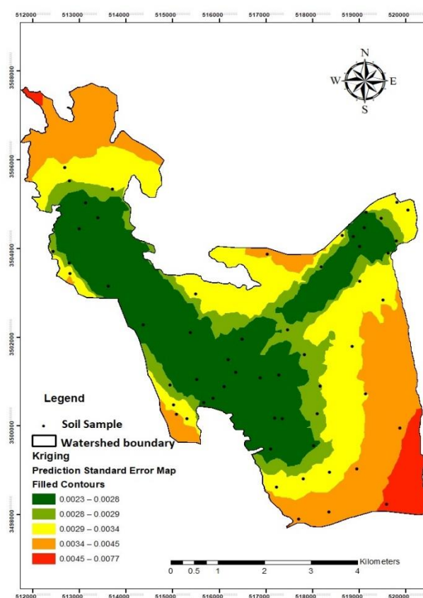
شکل ۶: نقشه‌ی خطای تخمین روش کریجینگ معمولی
