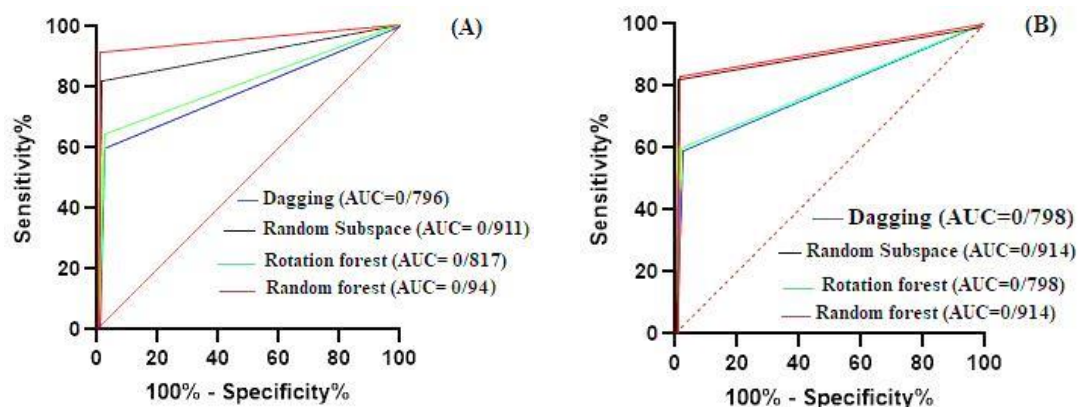
شکل ۷: منحنی ROC برای نتایج الگوریتم های داده کاوی (A: آموزشی و B: اعتبارسنجی)
