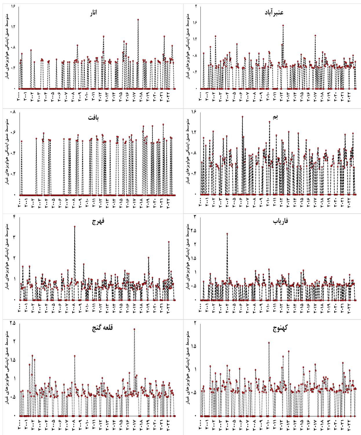
شکل ۳: تغییرات متوسط ماهانه عمق ایتیکی هوایزها در مناطق مختلف استان کرمان طی بازه زمانی (۲۰۰۰-۲۰۲۲)
