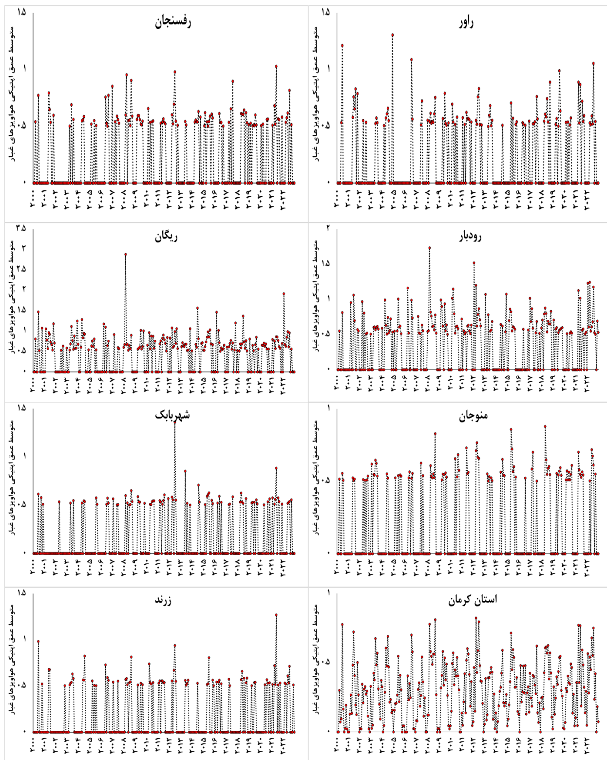
شکل ۵: تغییرات متوسط ماهانه عمق اینتیکی هواویزها در مناطق مختلف استان کرمان طی بازه زمانی (۲۰۰۰-۲۰۲۲)
