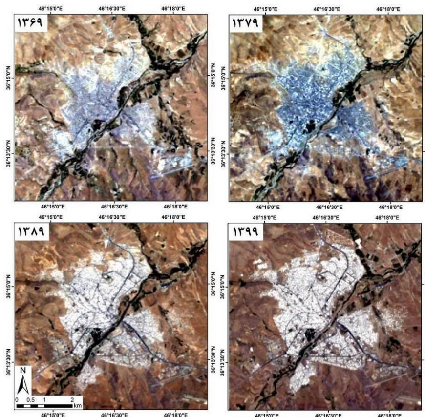
شکل ۴: تصاویر ماهواره نلدست مورد استفاده
