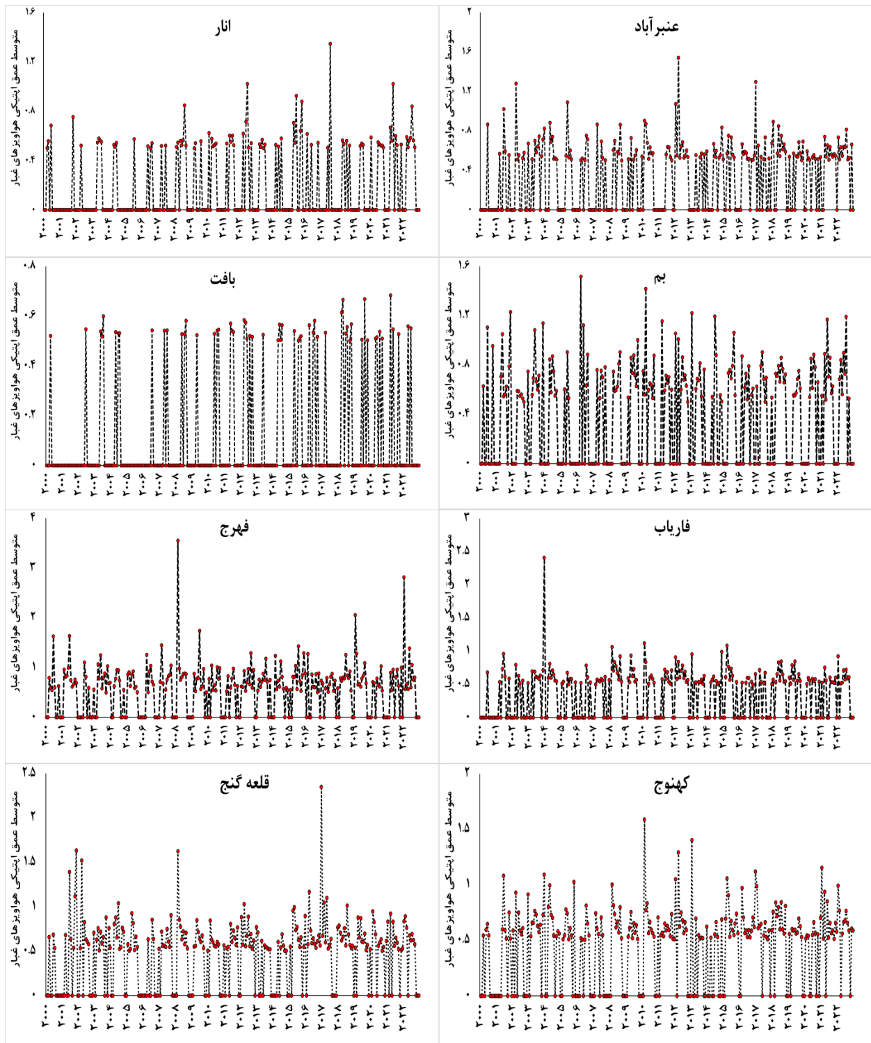
شکل ۳: تغییرات متوسط ماهانه عمق اینتیکی هواویزها در مناطق مختلف استان کرمان طی بازه زمانی (۲۰۰۰-۲۰۲۲)
