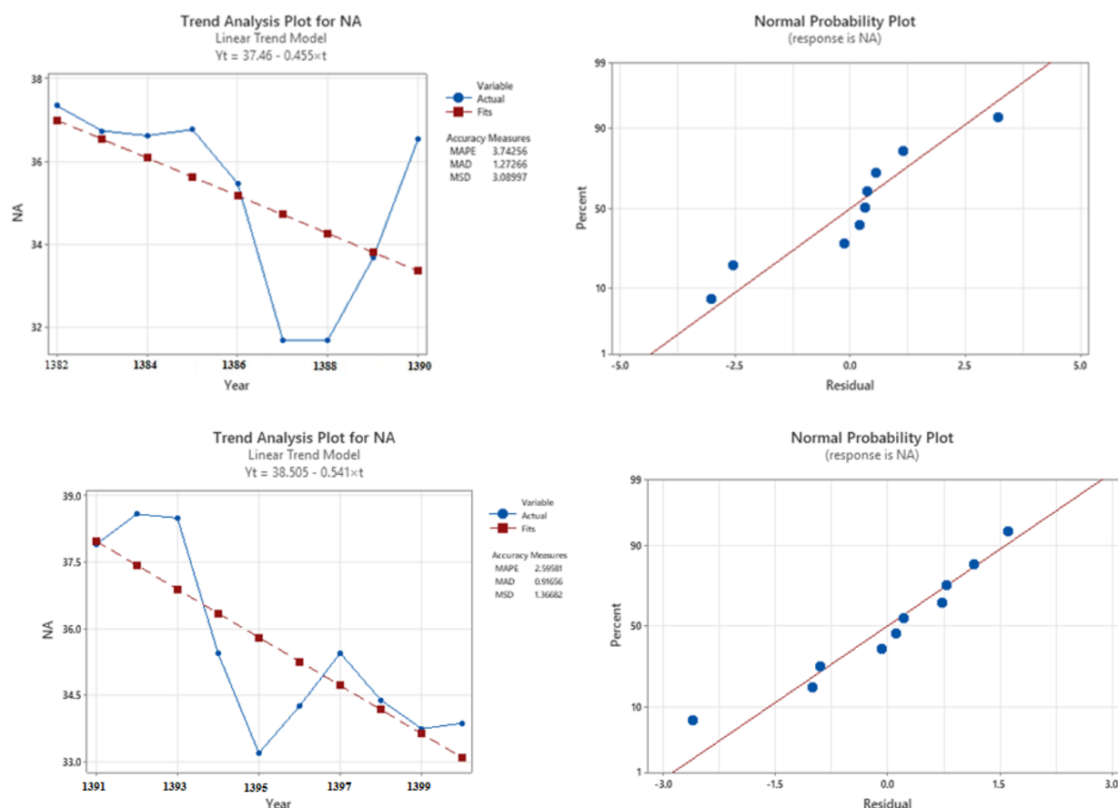
شکل ۸: آنالیز روند خطی میانگین Na در دوره‌های اول (۱۳۸۲-۱۳۹۰) و دوم (۱۳۹۱-۱۴۰۰)
