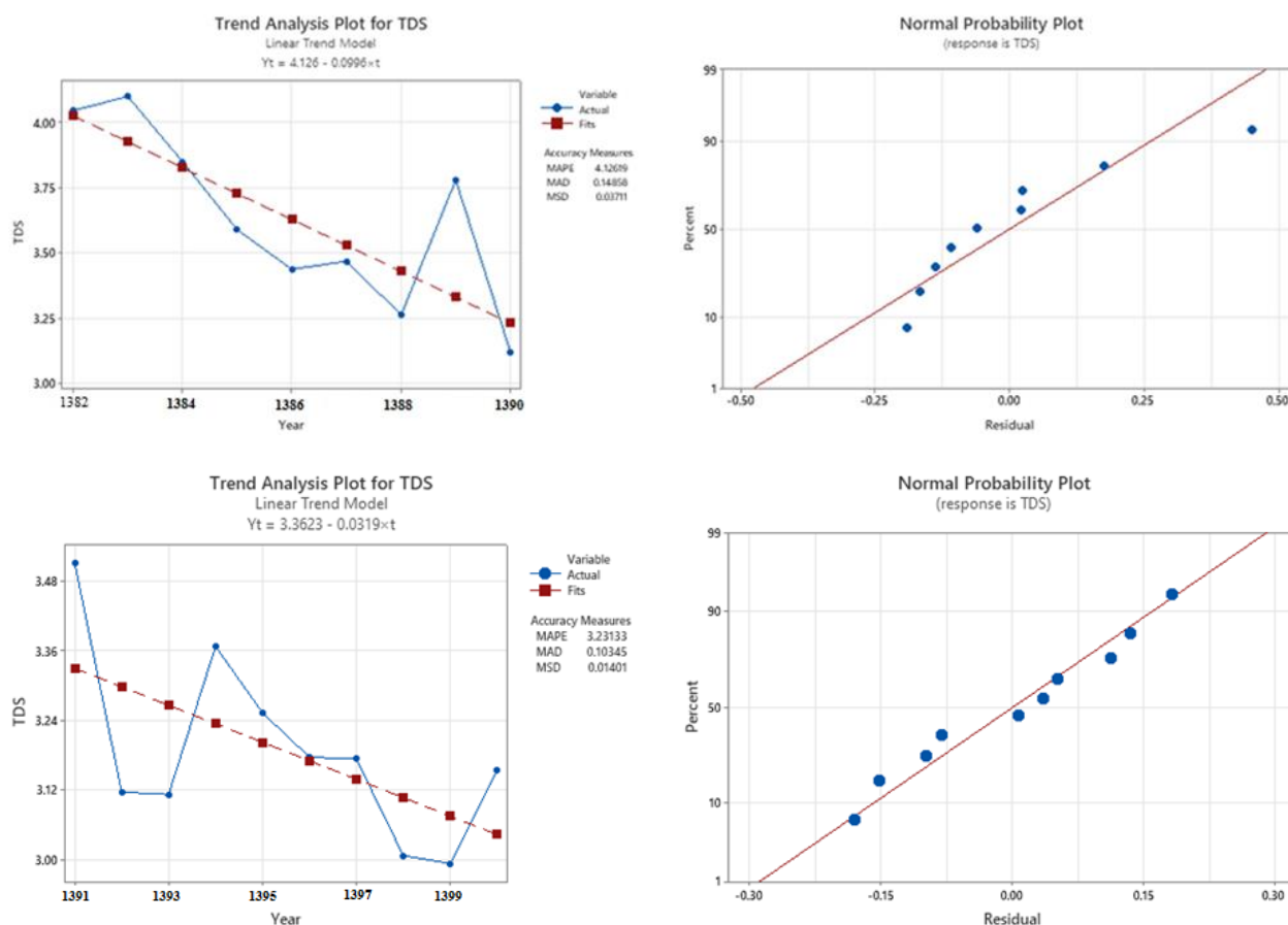
شکل ۳: آنالیز روند خطی میانگین TDS در دوره‌های اول (۱۳۸۲-۱۳۹۰) و دوم (۱۳۹۱-۱۴۰۰)
