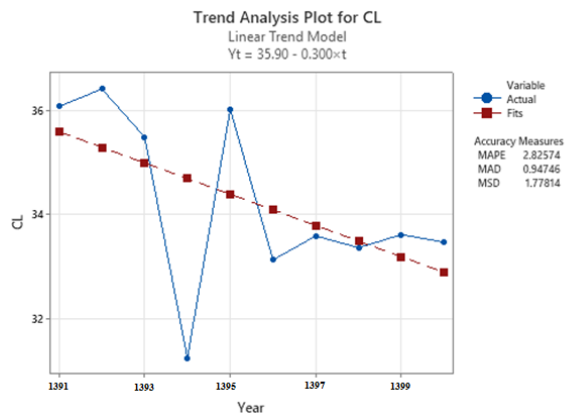
شکل ۴: آنالیز روند خطی میانگین CL در دوره‌های اول (۱۳۸۲-۱۳۹۰) و دوم (۱۳۹۱-۱۴۰۰)
