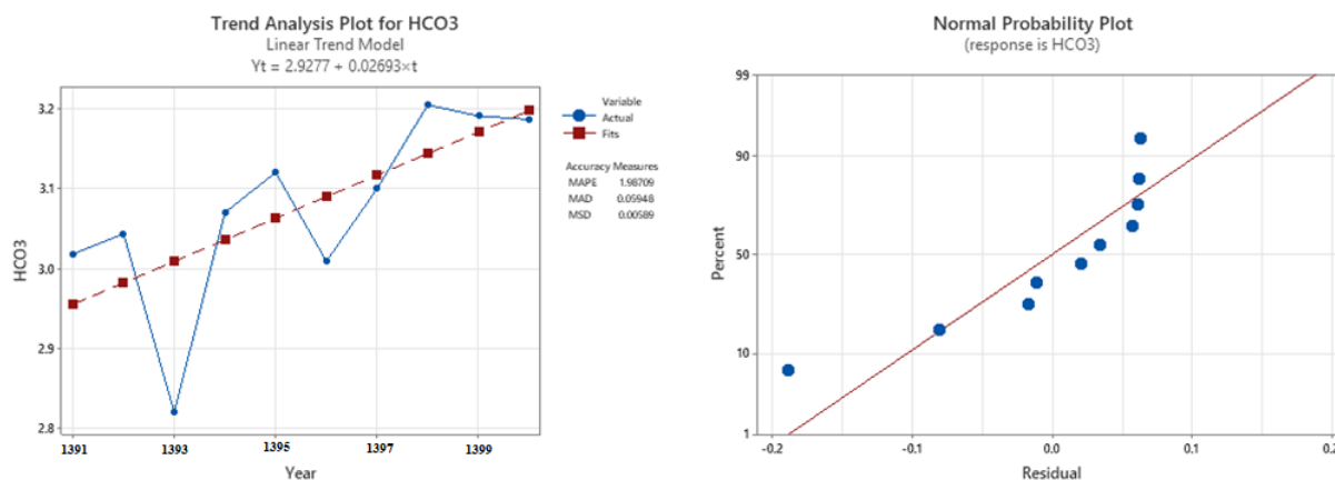
شکل ۷: آنالیز روند خطی میانگین HCO_3 در دوره‌های اول (۱۳۸۲-۱۳۹۰) و دوم (۱۳۹۱-۱۴۰۰)
