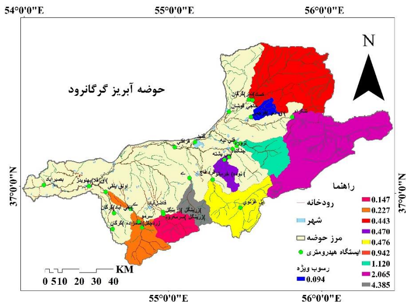
شکل ۸- نقشه رسوب ویژه حوضه آبریز گرگانرود
