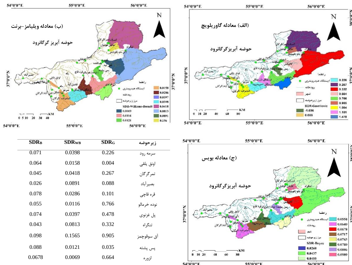
شکل ۶- نقشه‌های نسبت تحویل رسوب (SDR) زیرحوضه‌های مورد مطالعه که بر اساس سه معادله (الف) گاوریلویچ (SDR G ، (ب) ویلیامز-برنت (SDR B ) و (ج) بویس (SDR WB )
