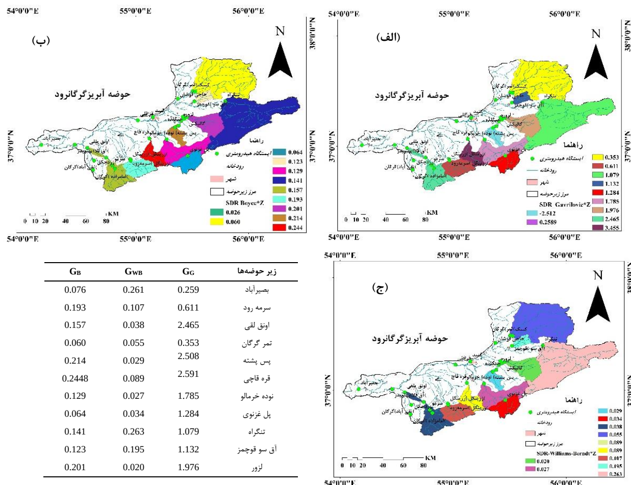
شکل ۷- نقشه بازده رسوب (G) در زیرحوضه‌های مورد مطالعه حوضه که توسط مدل EPM بر اساس معادله نسبت تحویل رسوب (الف) گاوریلیچ،
