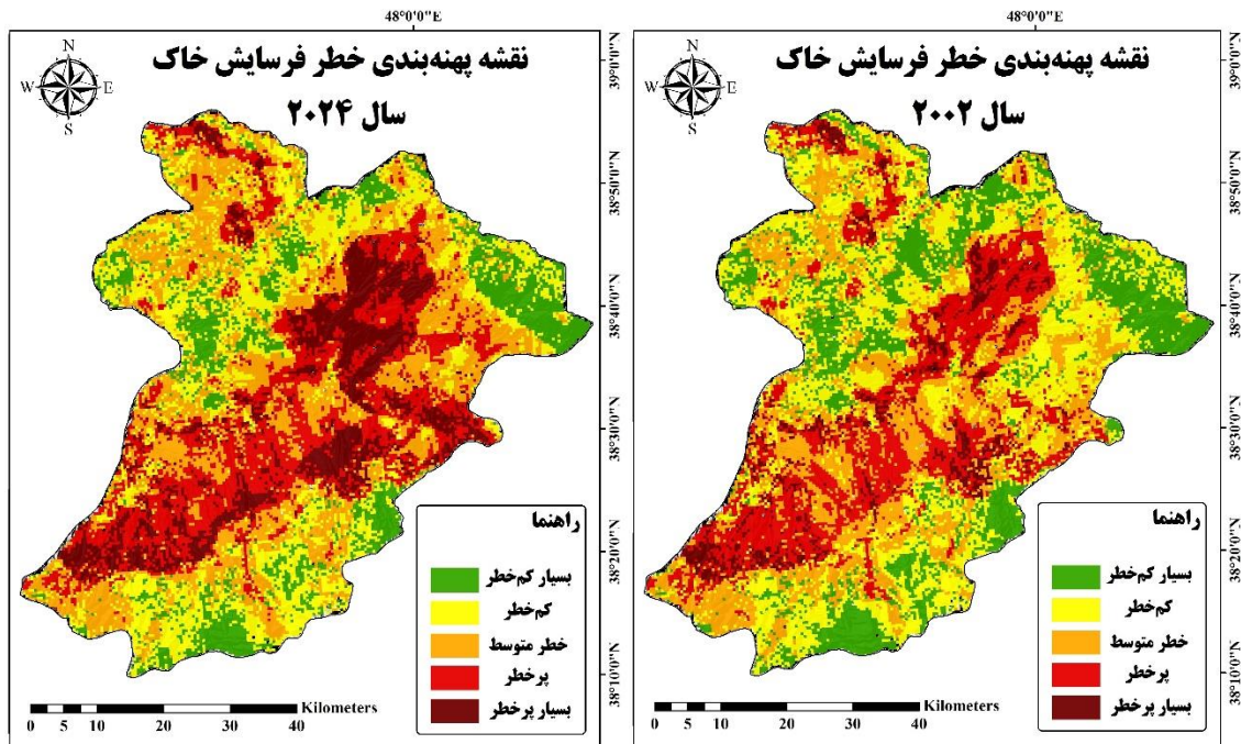
شکل ۸: نقشه پهنه‌بندی فرسایش سال ۲۰۲۴
