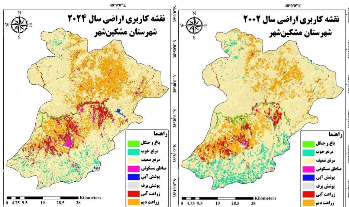
شکل ۴: نقشه کاربری اراضی سال ۲۰۰۲ شهرستان مشکین‌شهر
