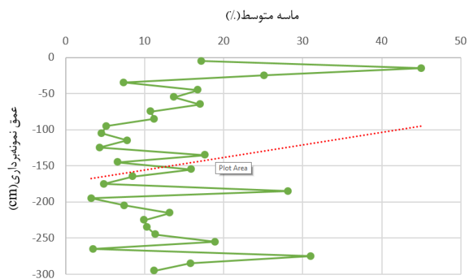
شکل شماره ۷: نمودار تغییرات سهم نسبی ماده متوسط نمونه‌های رسوب در اعماق مختلف نمونه‌برداری
