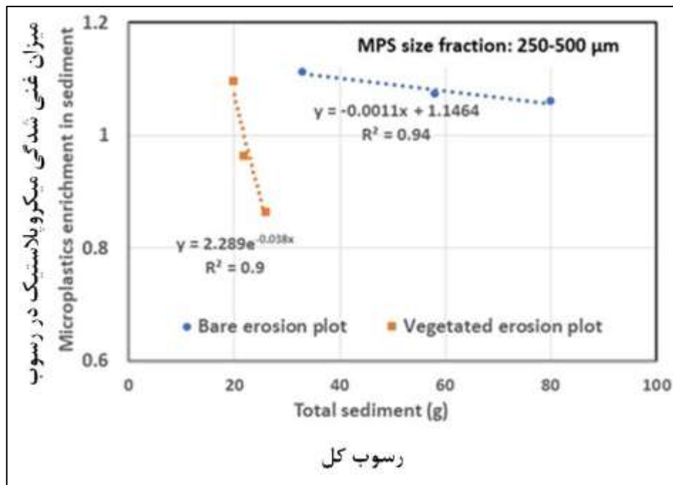
شکل ۵- ارتباط بین نسبت غنی شدگی میکروپلاستیک با رسوب کل خروجی از کرت فرسایشی.
